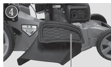
排出口カバーをかぶせる
