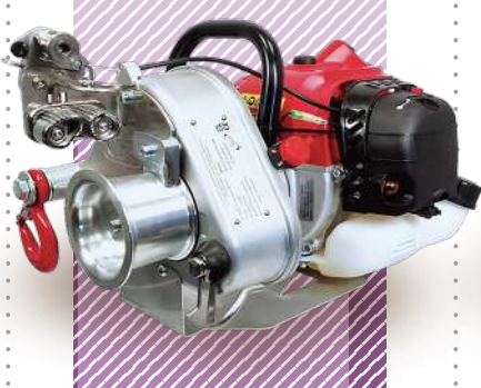
牽引用ロープウインチ 本体 NEW PCW4500 2サイクルエンジン式
